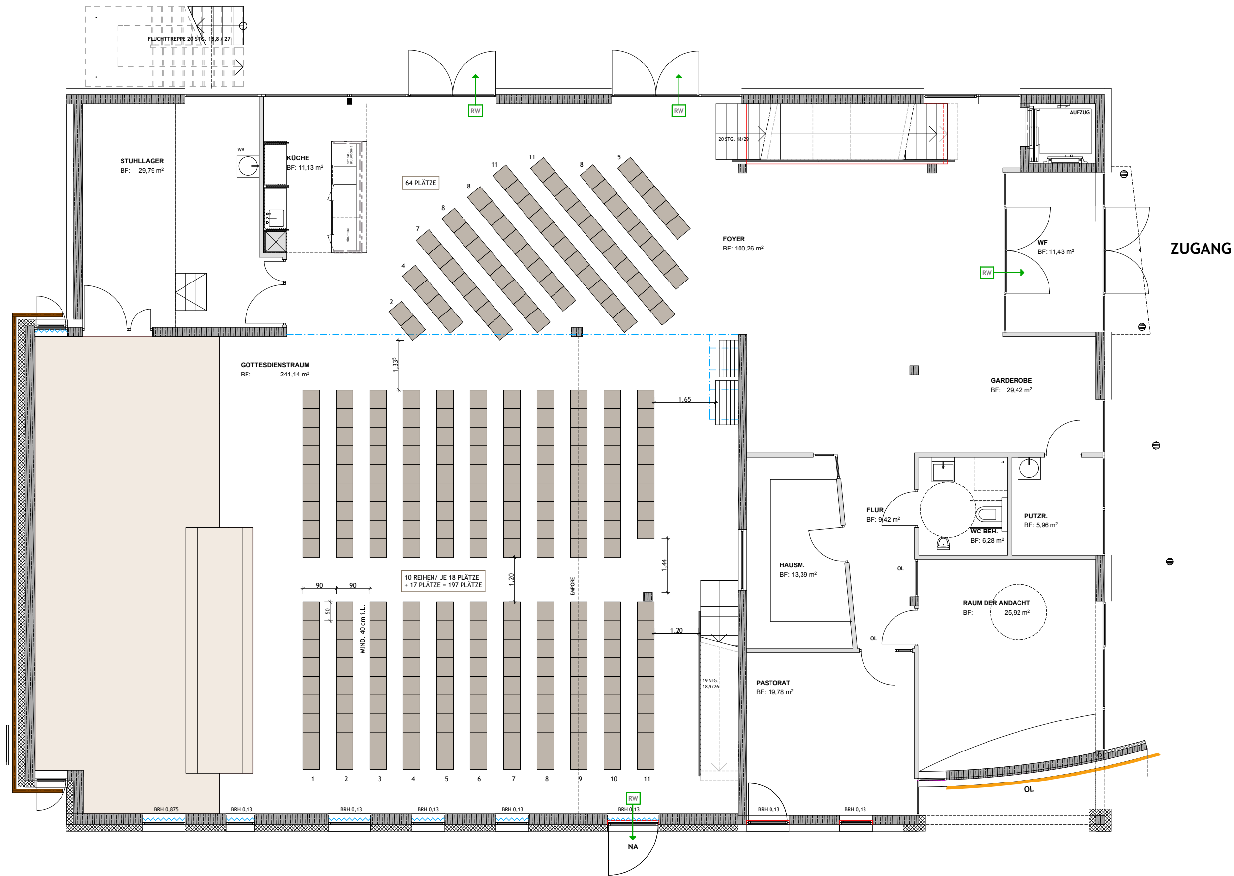
GOTTESDIENSTRAUM ERDGESCHOSS
